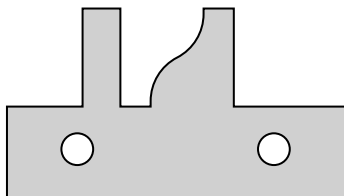
Profil 09.27701 (eingebaut)
